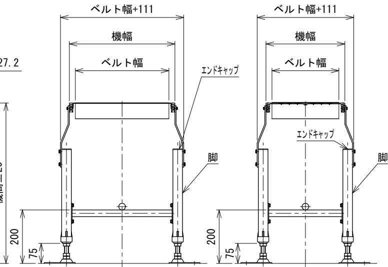
中間断面図(ベルト幅350~500 mm) 中間断面図(ベルト幅250・300 mm)
