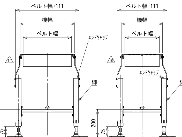
中間断面図(ベルト幅350~500 mm)
