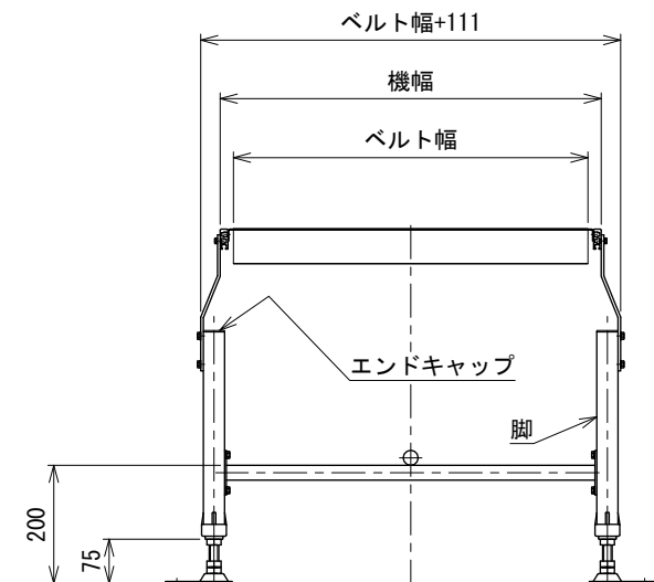
中間断面図
