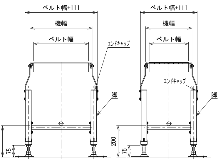
中間断面図(ベルト幅350~500 mm) 中間断面図(ベルト幅250・300 mm)
