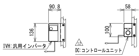
モーター関連寸法表 単位 mm
