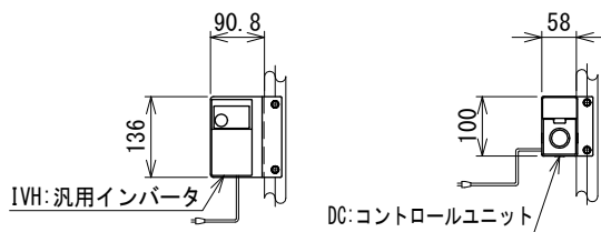
モータ関連寸法表 単位 mm
