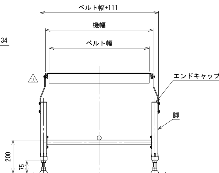
中間断面図
