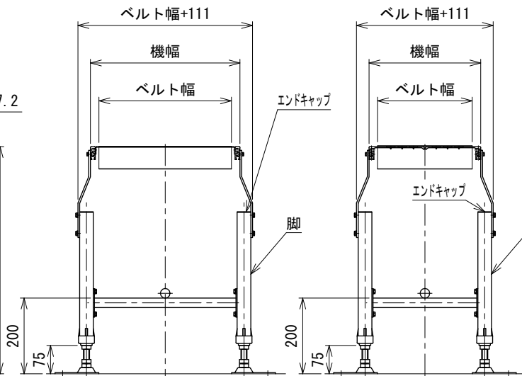
中間断面図(ベルト幅350~500 mm)
