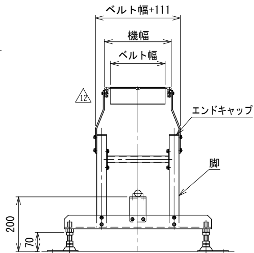
中間断面図
