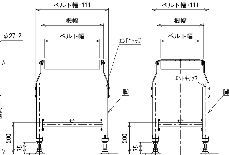
中間断面図 (ベルト幅350~500 mm) 中間断面図 (ベルト幅250・300 mm)
