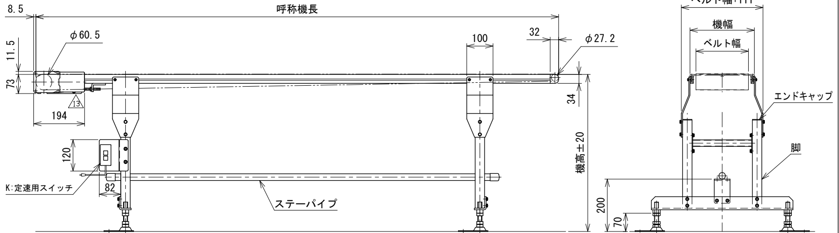
中間断面図
