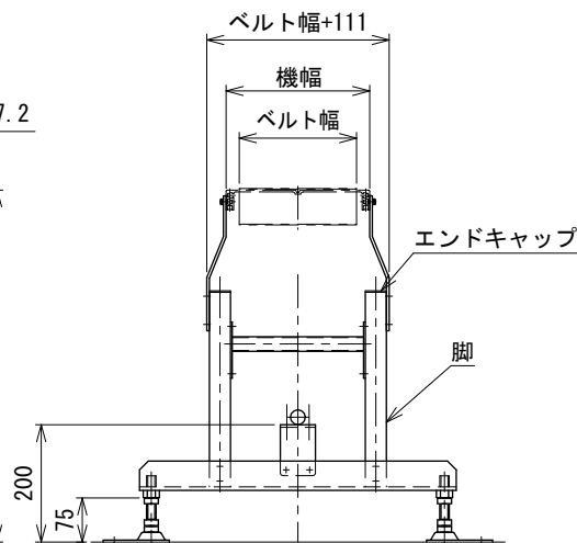
中間断面図
