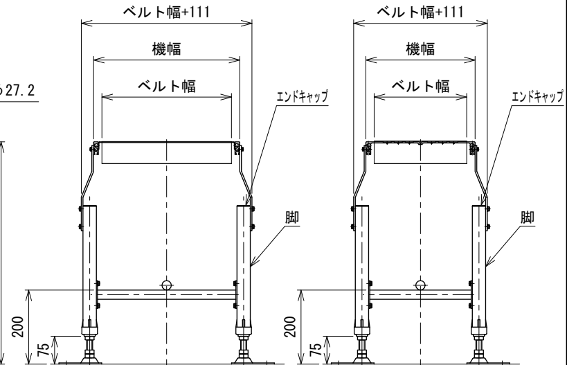
中間断面図(ベルト幅350~500 mm)
