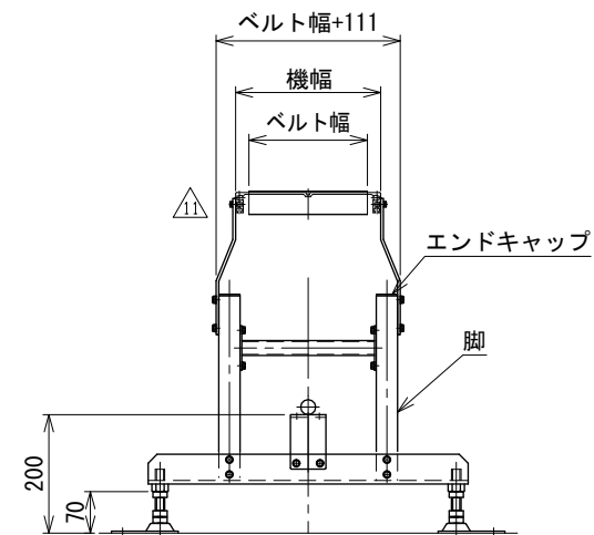
中間断面図
