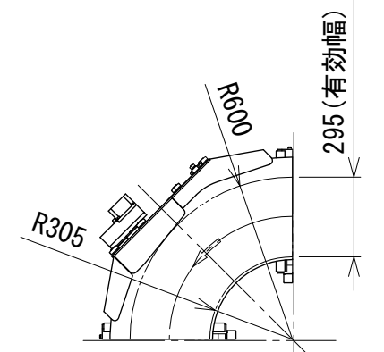
スパイラルカーブユニット詳細図
