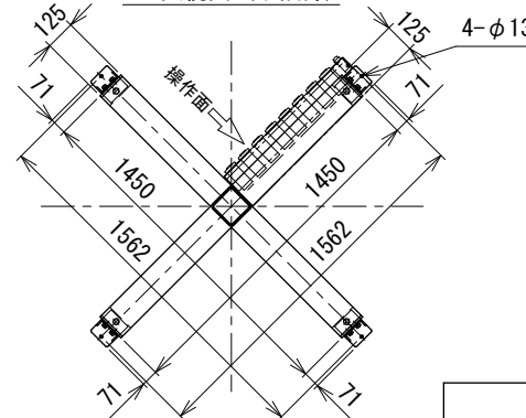
D-D矢視図
