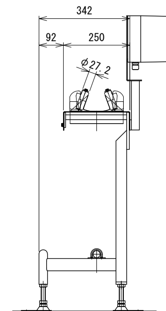
中間断面図
