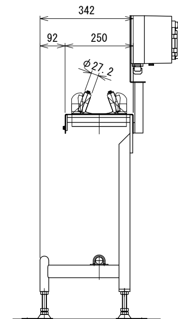
中間断面図
