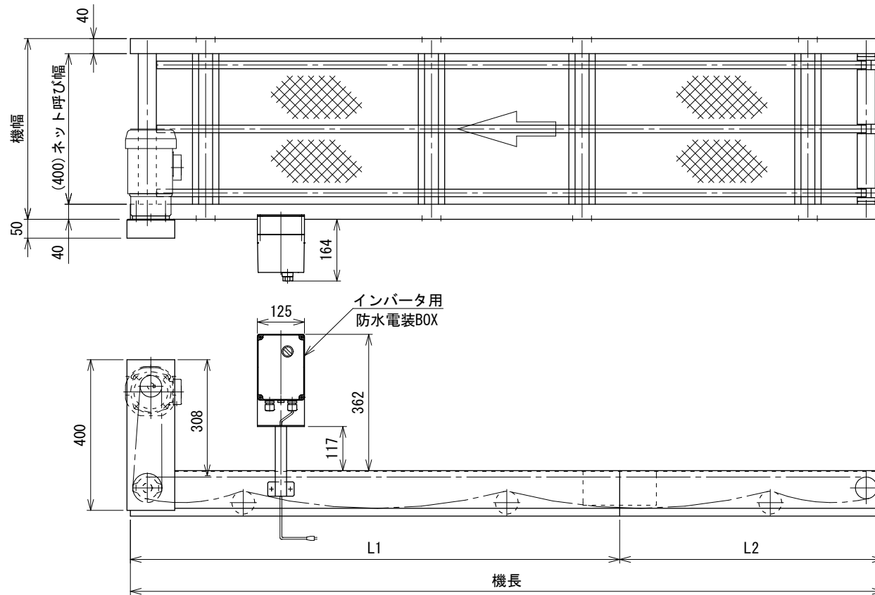
フレーム分割寸法
