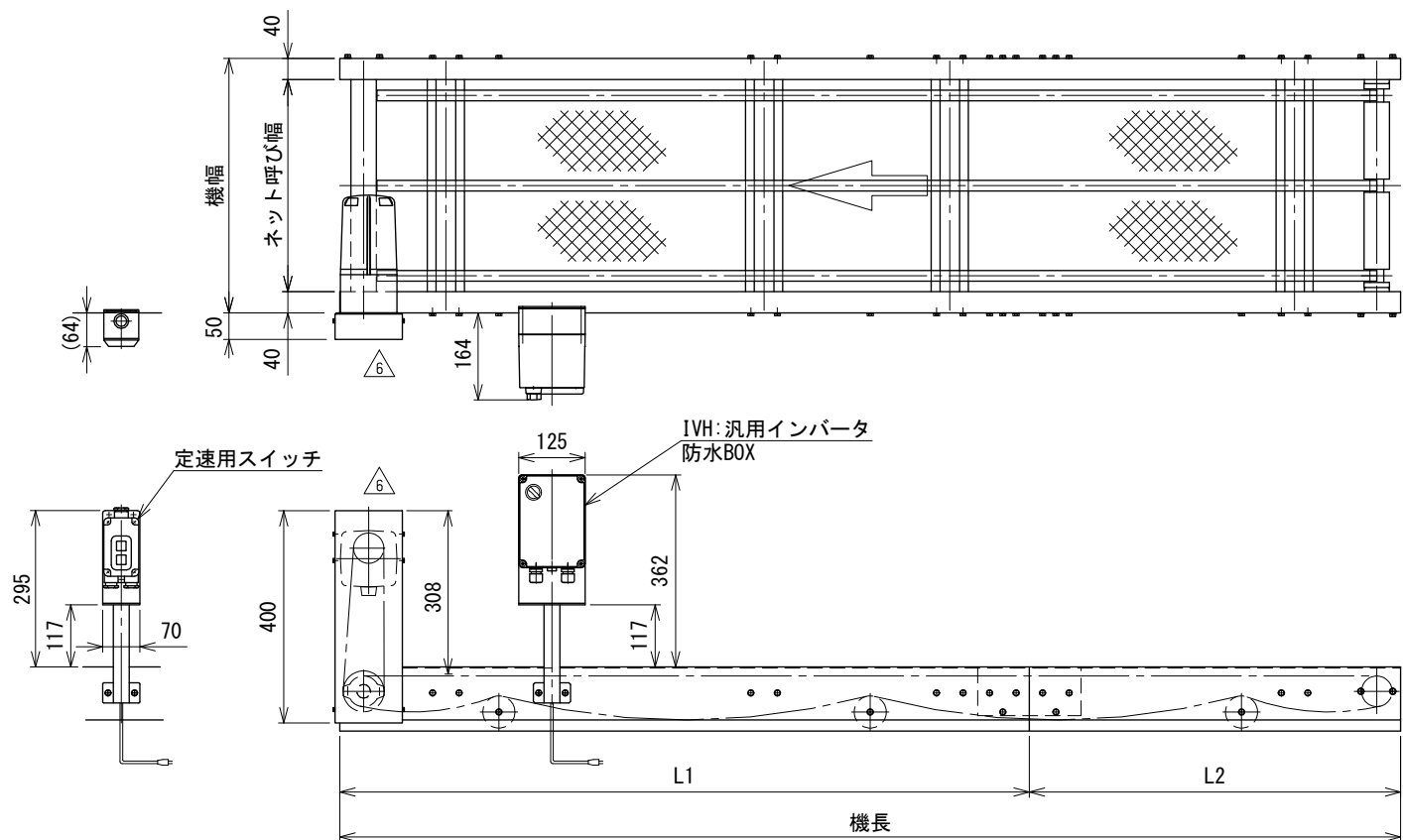
フレーム分割寸法
