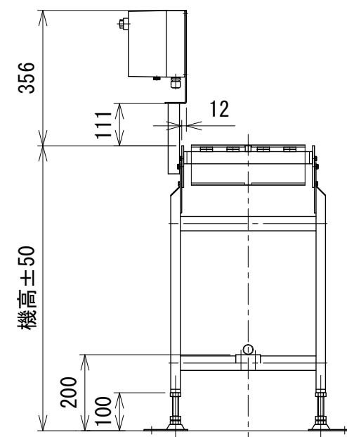
中間断面図
