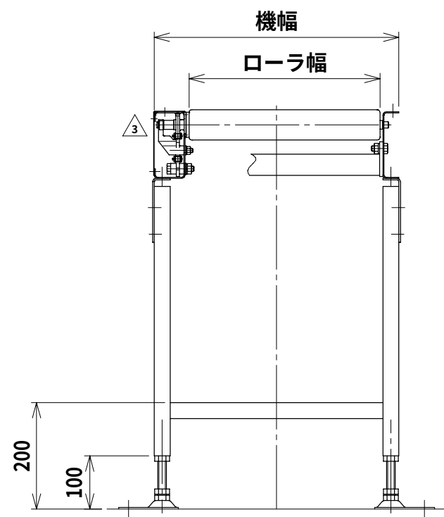
中間断面図
