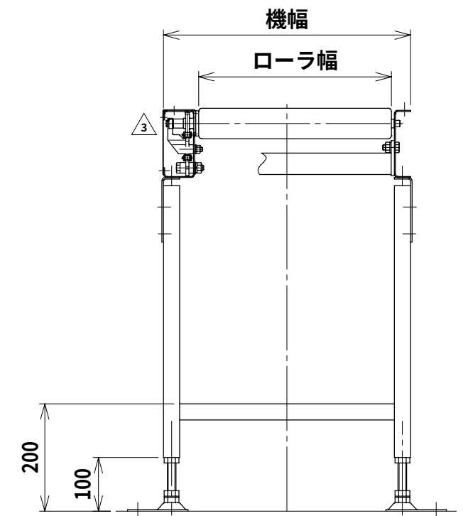
中間断面図
