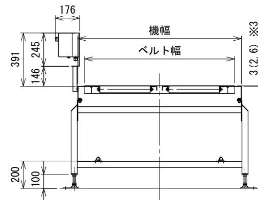
中間断面図
