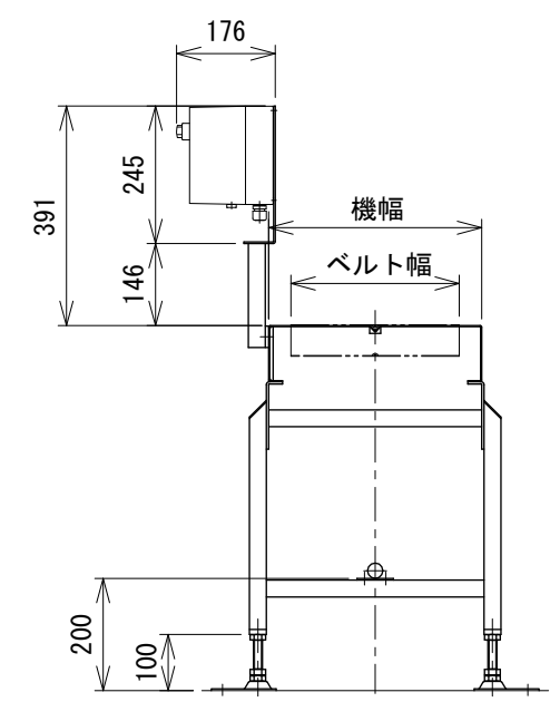
中間断面図
