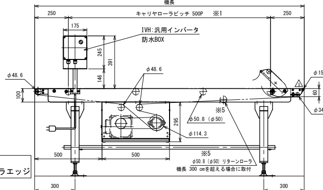
REBL3 両側ローラエッジ
