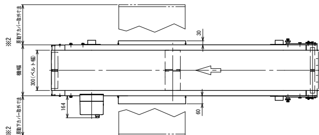
REBL1 出口側ローラエッジ
