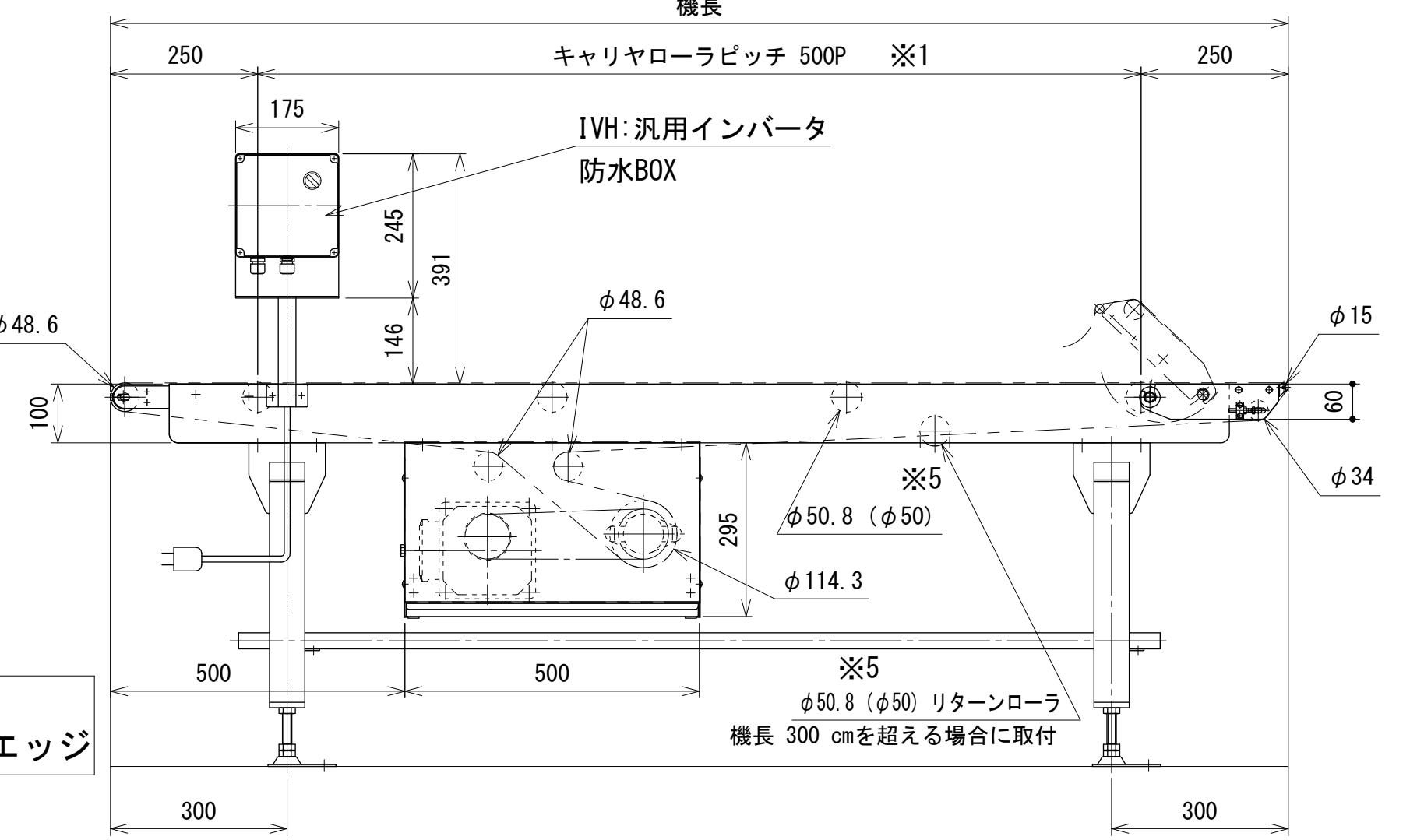
REBL3 両側ローラエッジ
