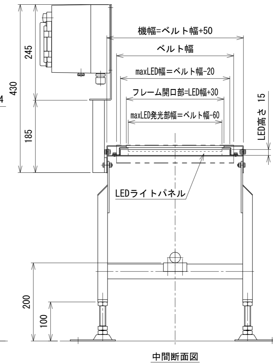
ルーバ付き電源ボックス取付け図 ※1 ※2 タイプC
