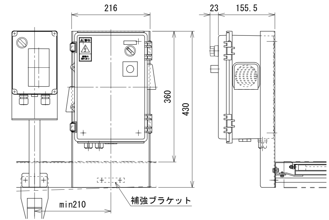
ルーバ付き電源ボックス取付け図 ※1 ※2 タイプC
