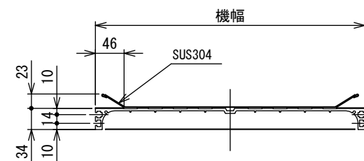
中間断面図
