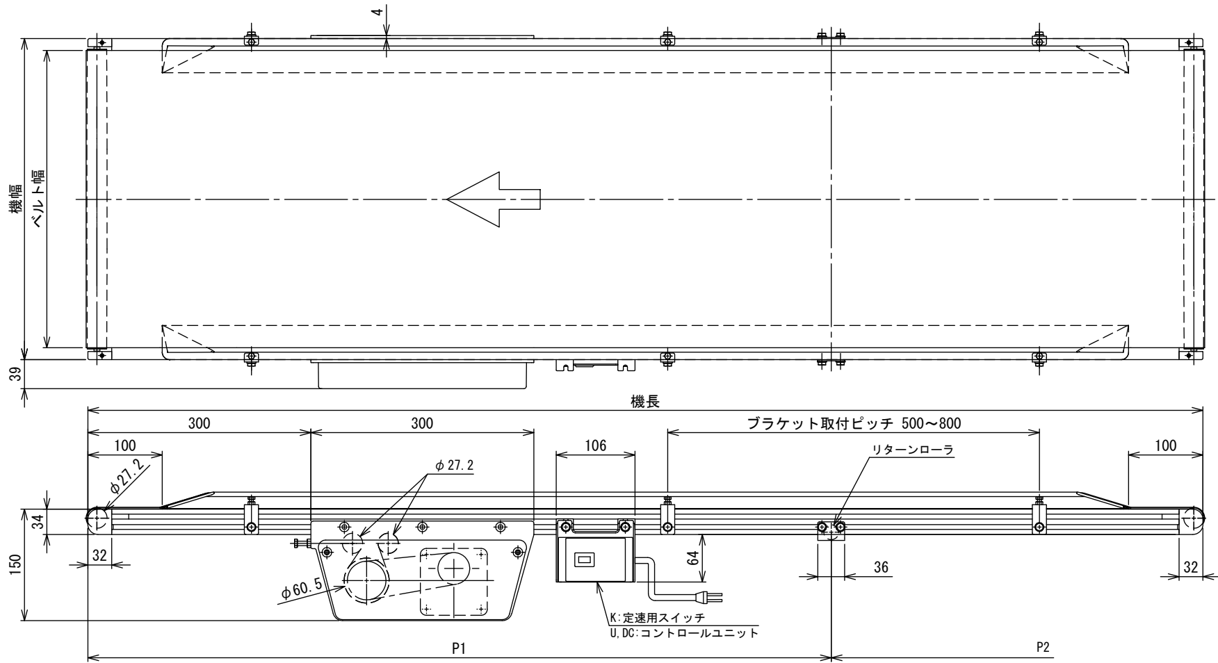
リターンローラ取付寸法表 単位mm
