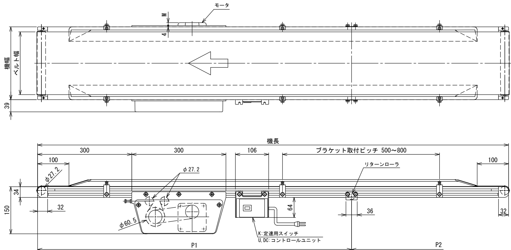
モーター飛び出し寸法表 M(最大値) 単位mm
