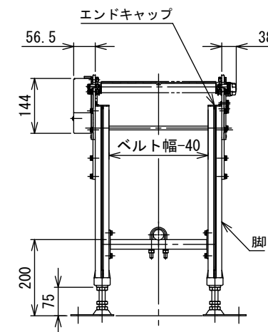
中間断面図
