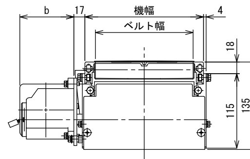
中間断面図
