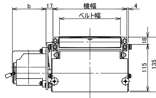
中間断面図
