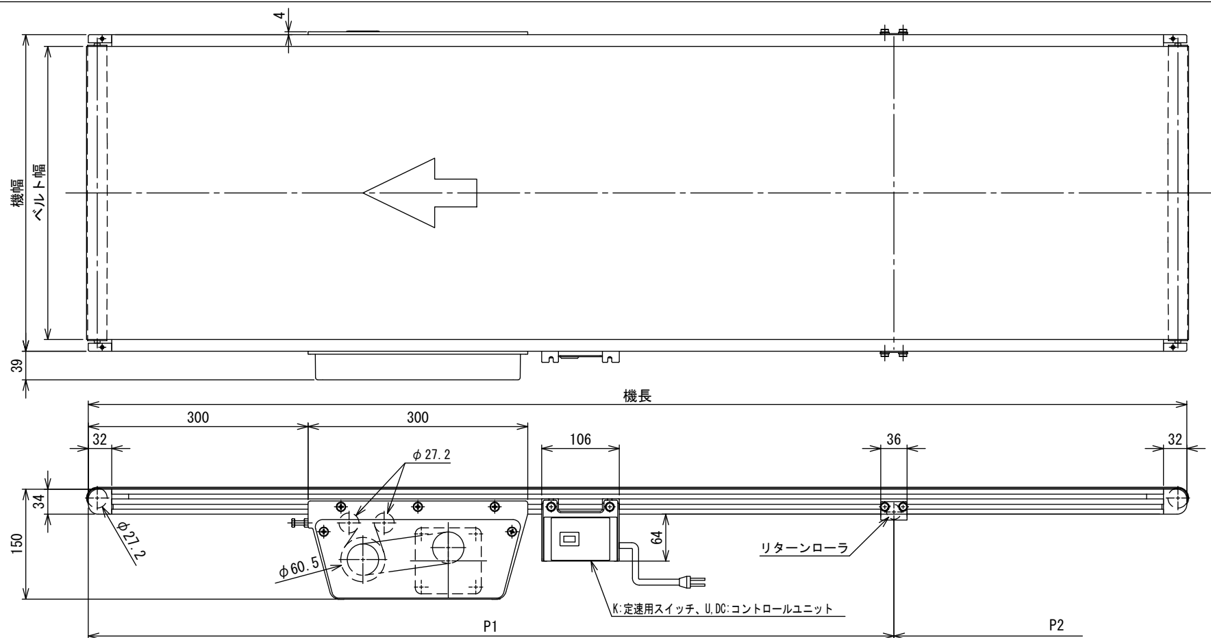
リターンローラ取付寸法表 単位:mm
