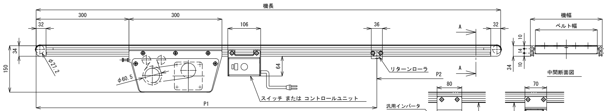
モータ飛び出し寸法表 M(最大値) 単位 mm
